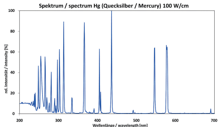
UVATEC Standardspektrum
